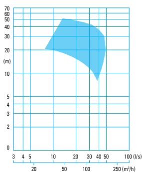
CMX 13... -2 pole
