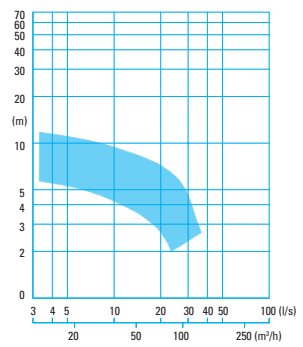
CMX 13... -4 pole
