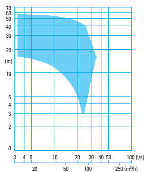
CV 13... -2 pole
