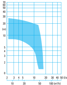
CTP... -2 + 4 pole
